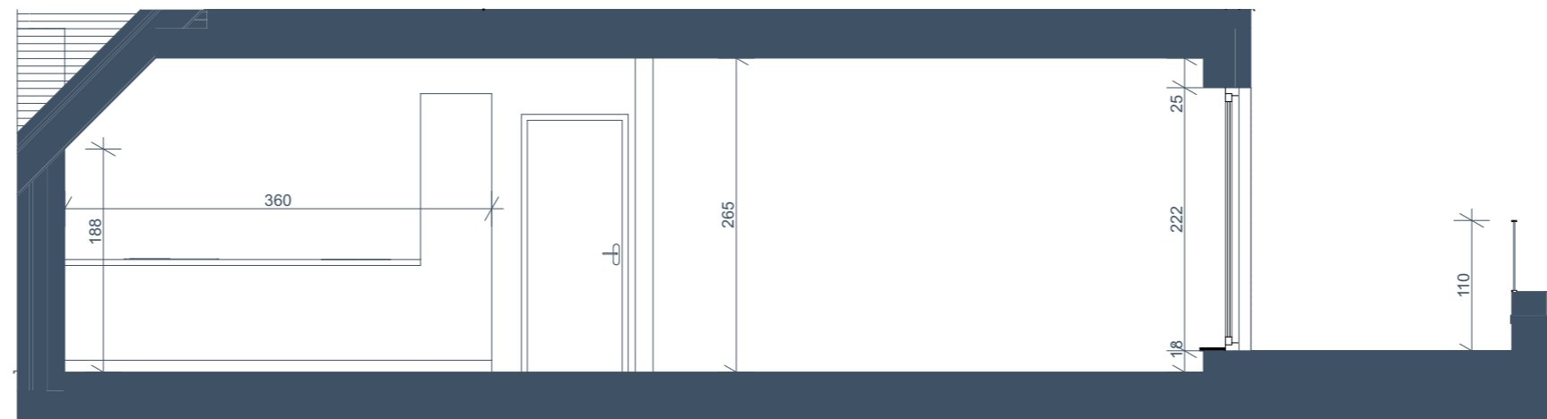
DOORSNEDE A
