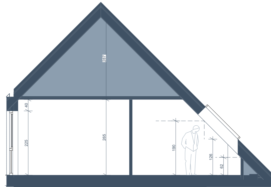
DOORSNEDE B
