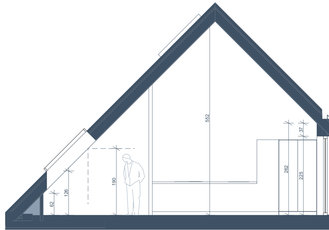
DOORSNEDE A
