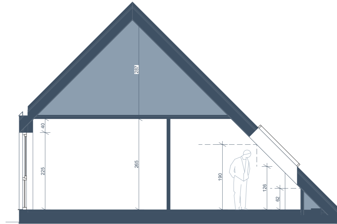
DOORSNEDE B
