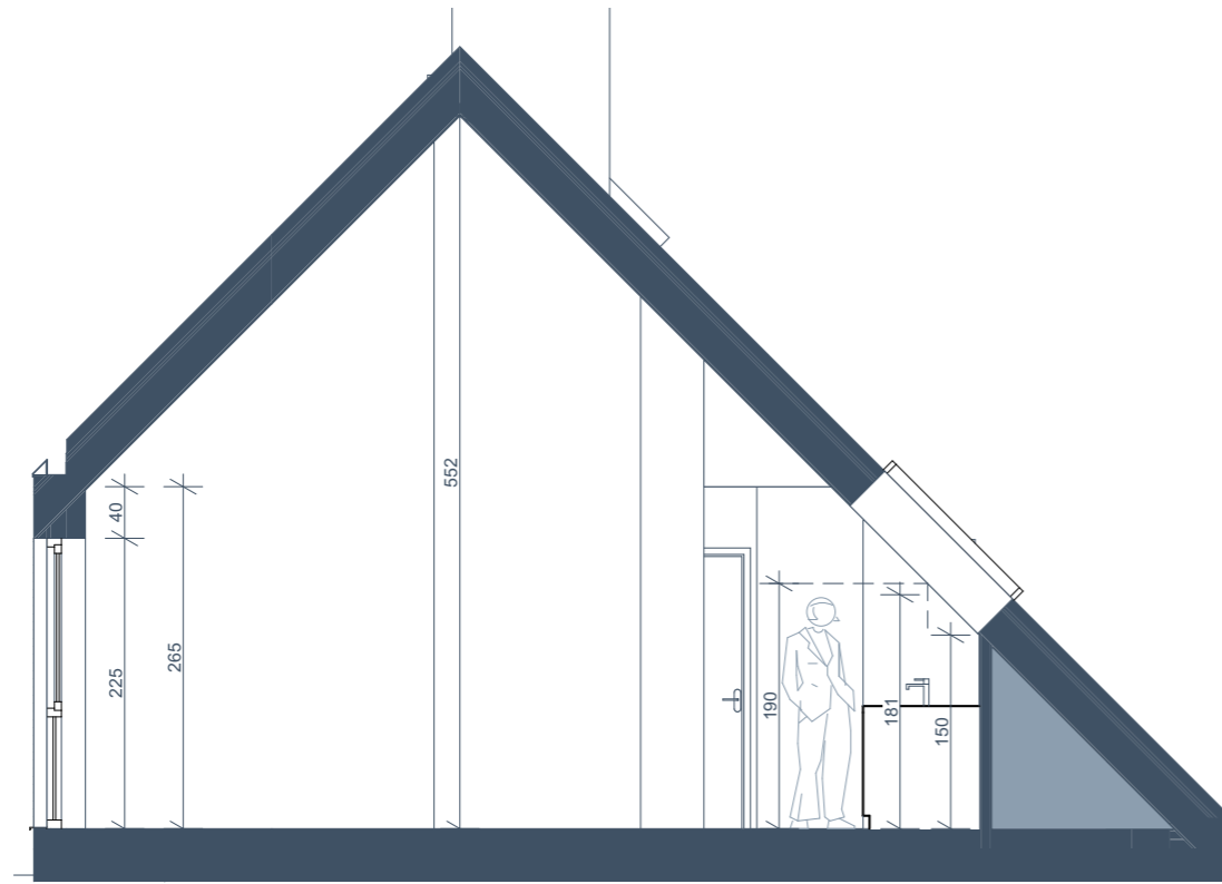
DOORSNEDE A
