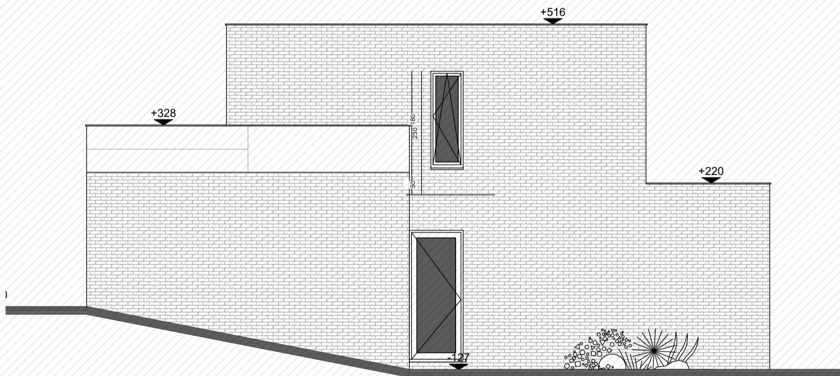
Zijgevel Rechts
