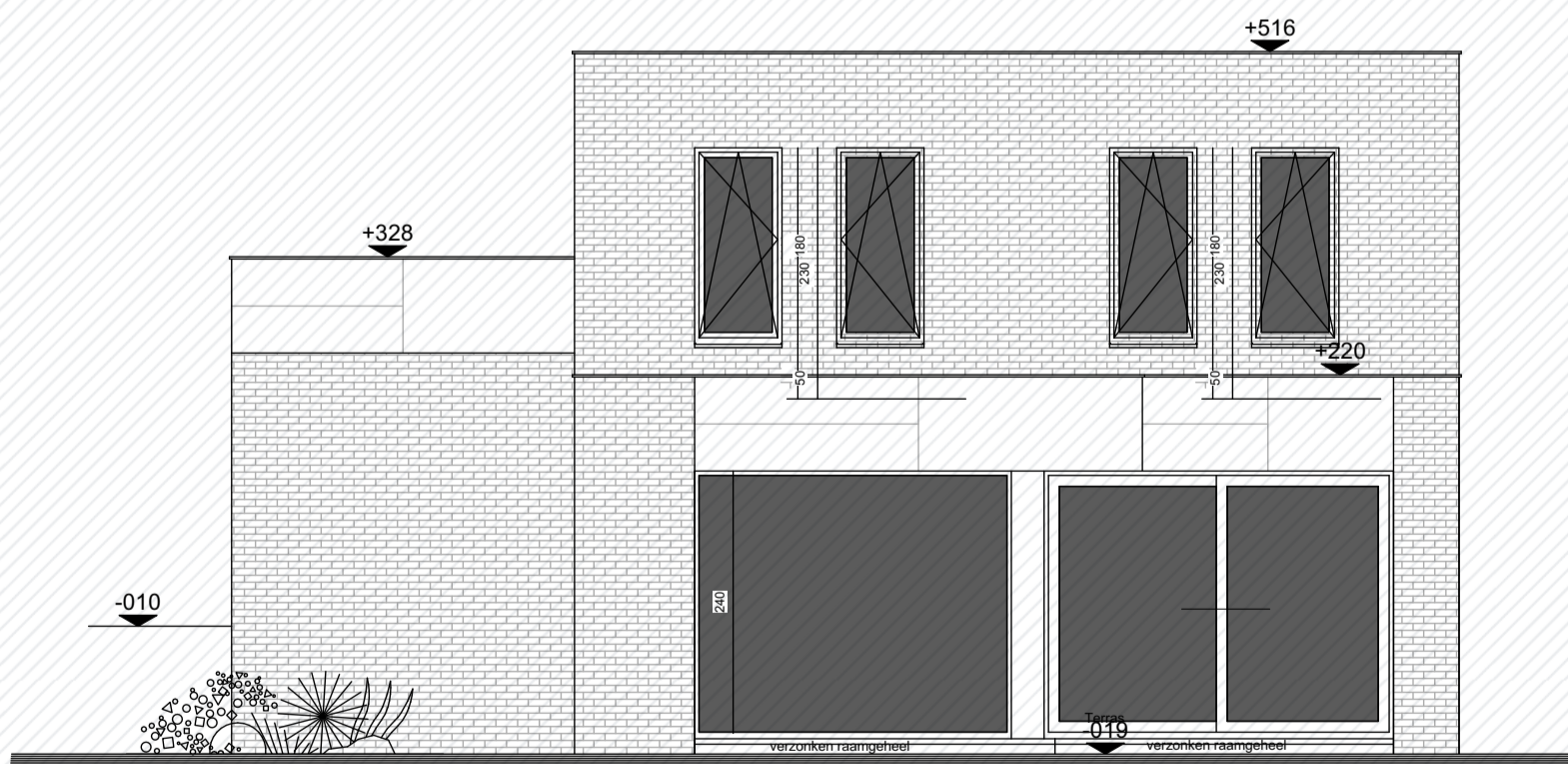
Achtergevel
