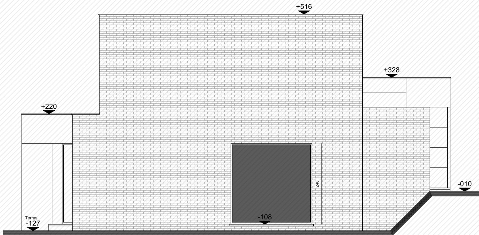
Zijgevel Links
