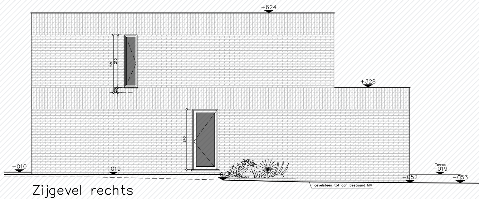
Achtergevel
